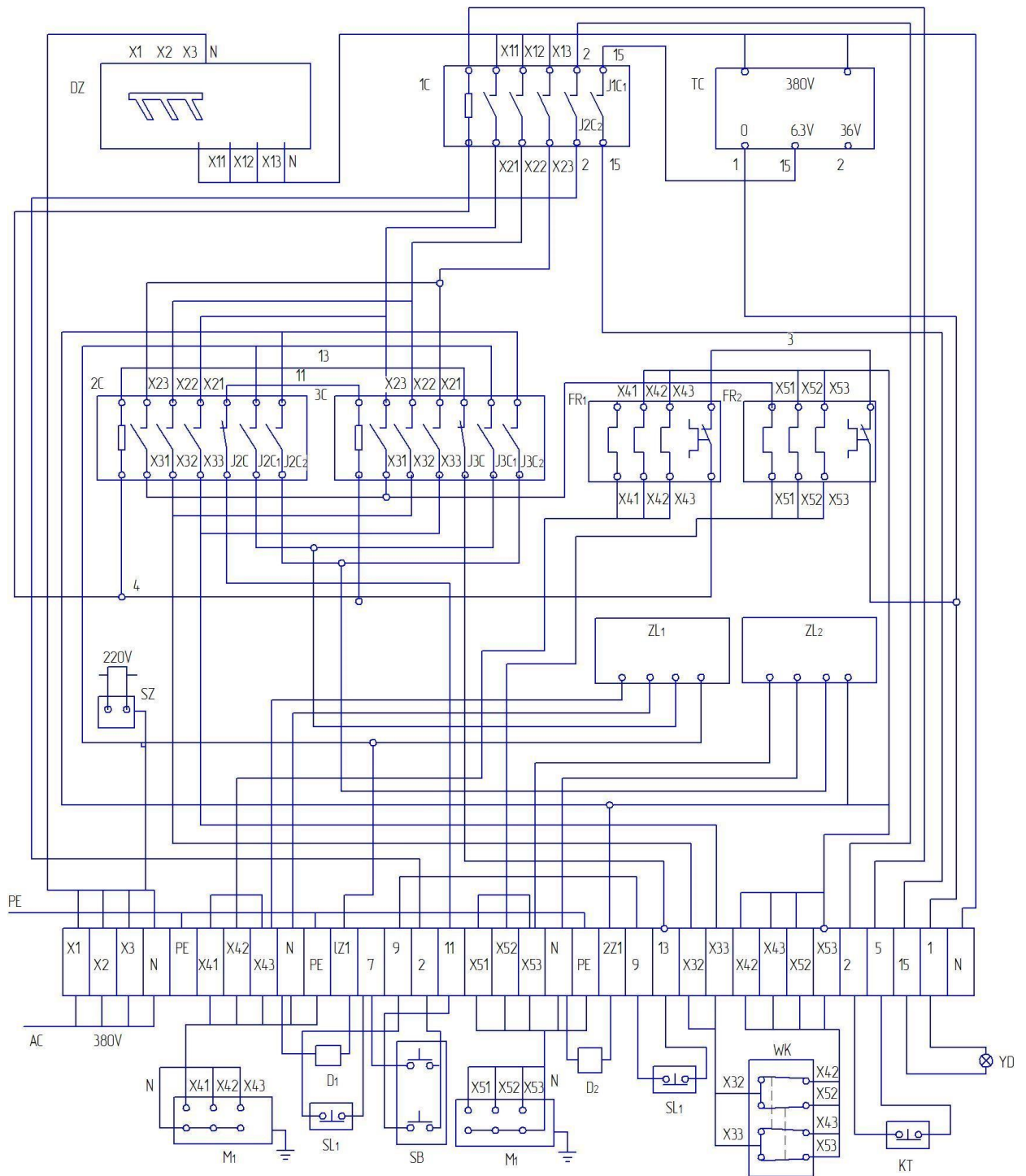
Рисунок 11 – Схема электрическая соединений
