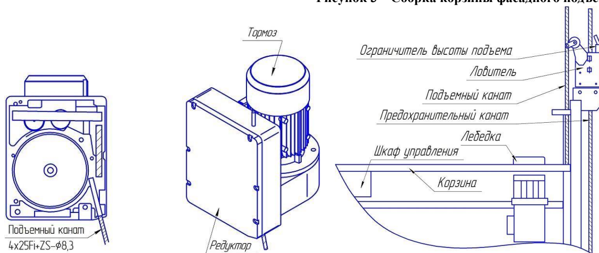
Рисунок 3 – Сборка корзины фасадного подъемника
