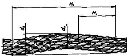
Рисунок 15 – Волнистость каната
